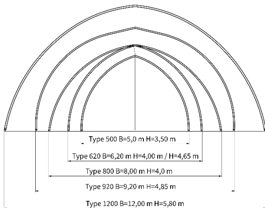
Verfügbare Spannweiten der AGROTEL Rundbogenhalle mit statischem Nachweis.
